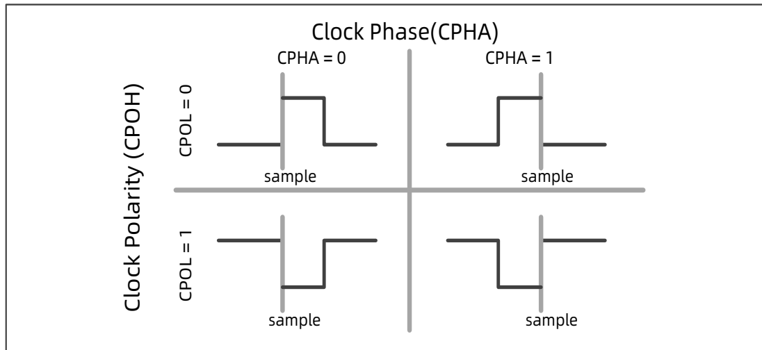
图 12.3 SPI 时钟格式图
