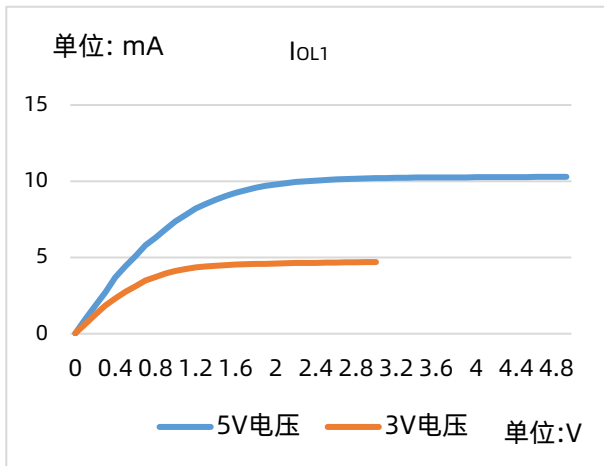
弱驱动模式下灌电流
