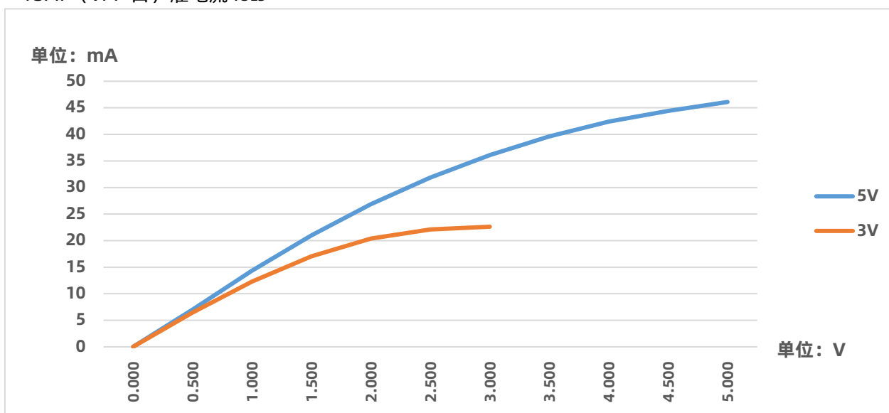
IOA7 (VPP 口) 灌电流 IOL3
