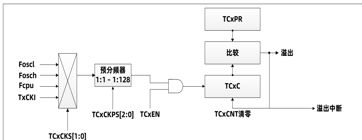
TC0/TC1 框图
