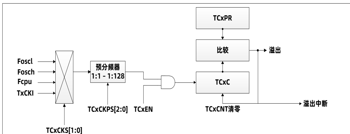
TC0/TC1 框图
