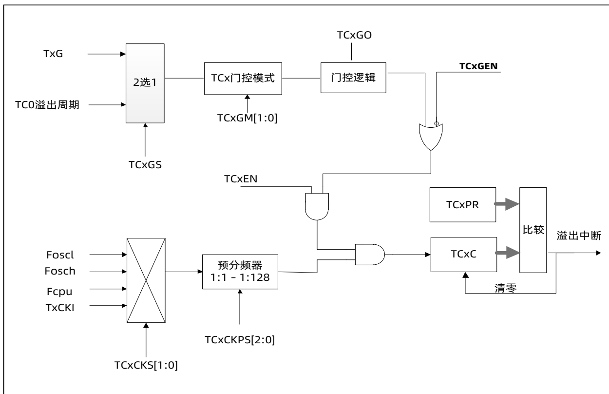
TCx(x=2、3、4)框图
