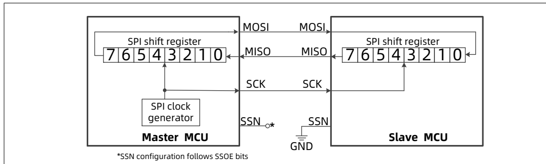
图 12.2-2 SPI 单主机单从机连接图
